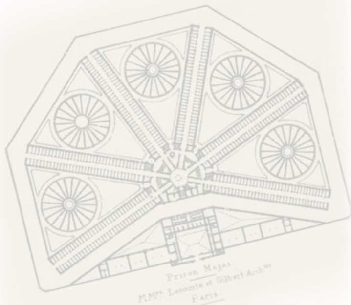
Plan de la prison de Mazas - 1836 (Coll. CRHCP)
