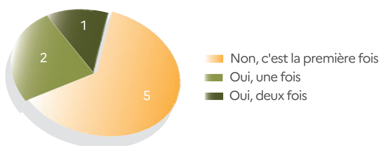
Graphique 5 : Aviez-vous déjà tenté le concours de directeur technique ? – Effectifs
