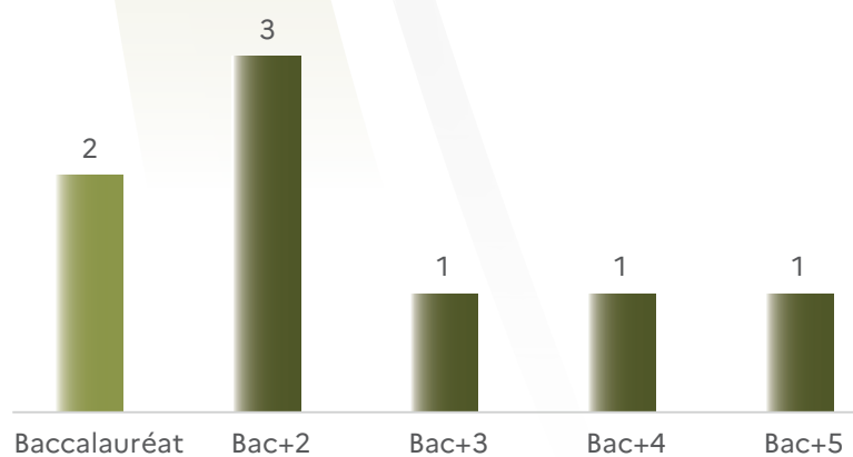
Graphique 3 : Diplôme le plus élevé obtenu – Effectifs
